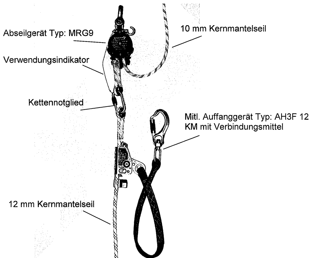
Bild 1: mitlaufendes Auffanggerät einschließlich beweglicher Führung Typ: FallArrescue
